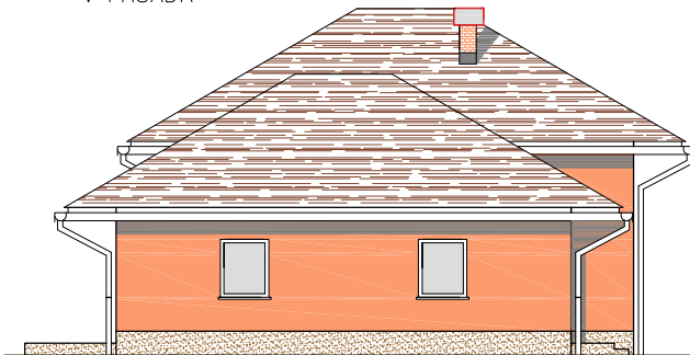
V FASADA
