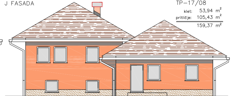
J FASADA
