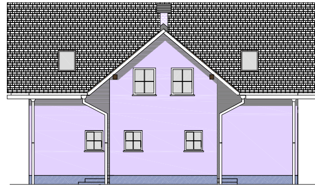
S FASADA
