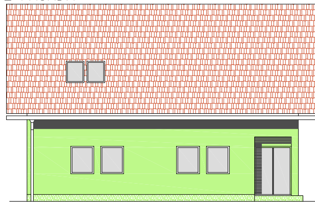
Z FASADA
