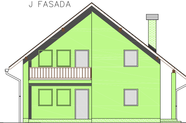
J FASADA
