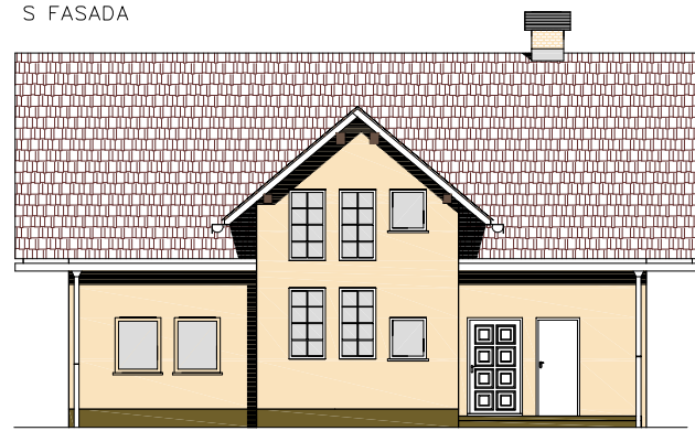
S FASADA
