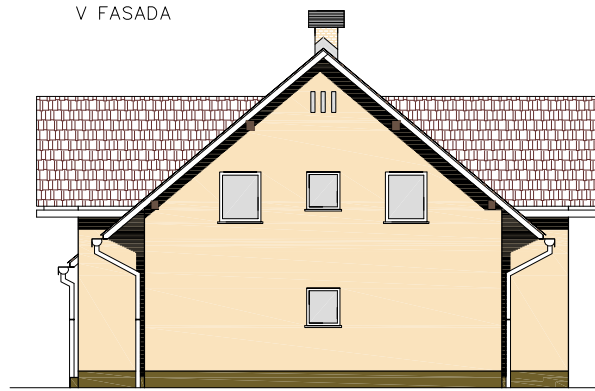
V FASADA
