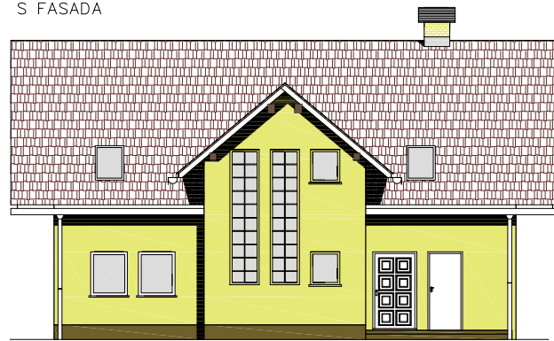
S FASADA
