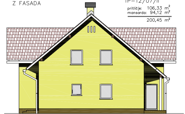
Z FASADA
