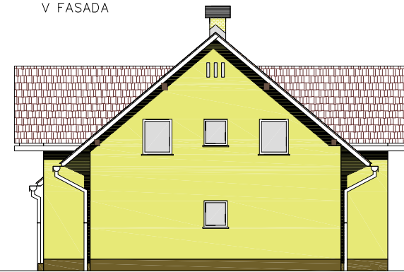
V FASADA
