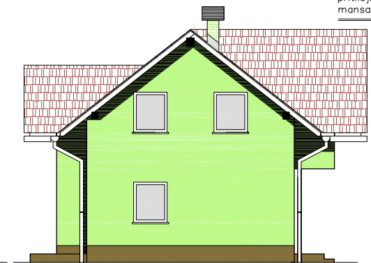
V FASADA
