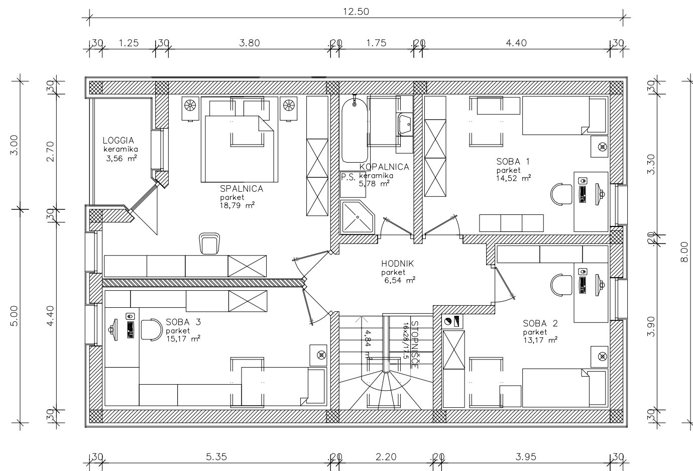
TLORIS MANSARDE
