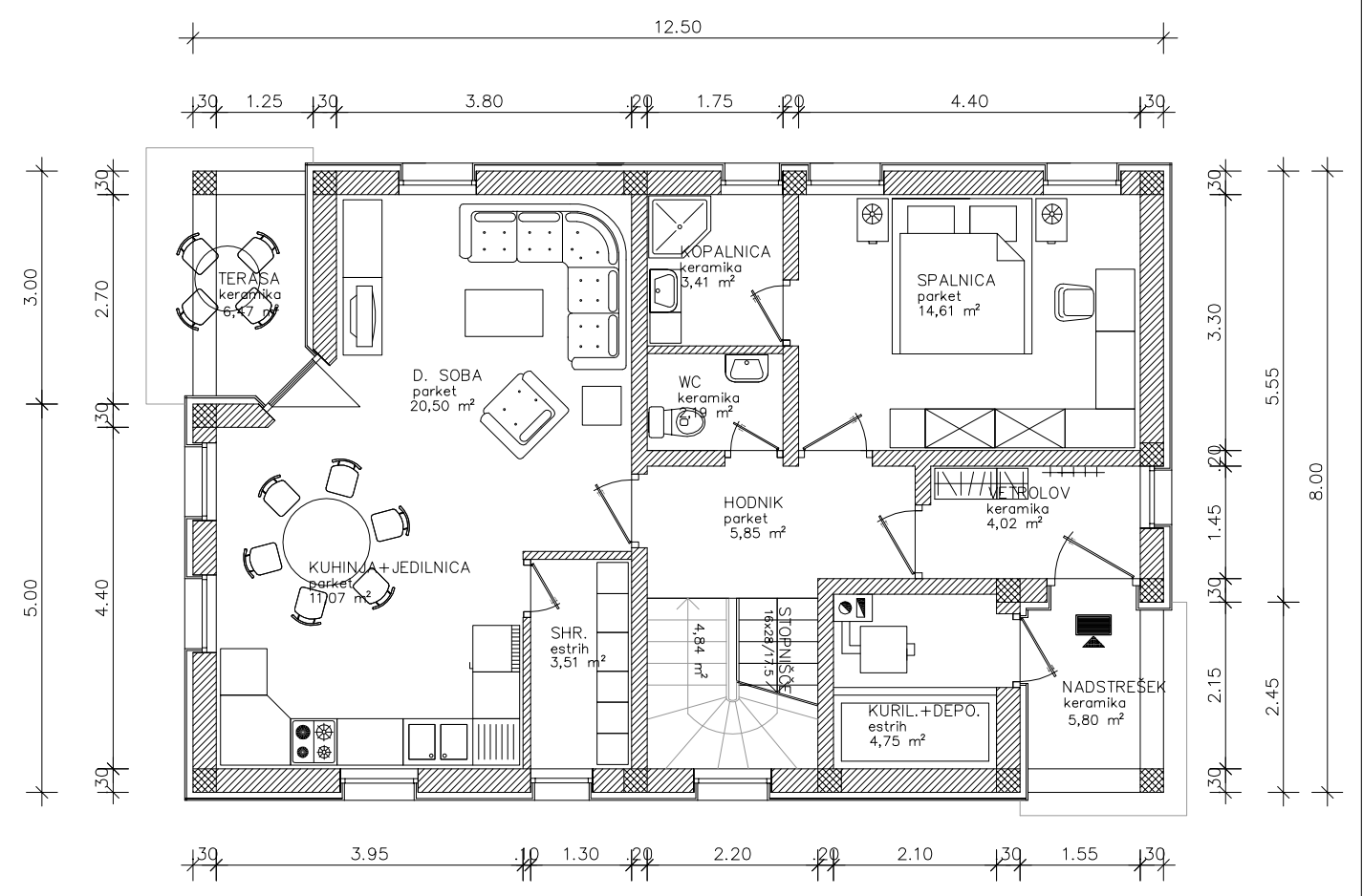
TLORIS PRITLIČJA
